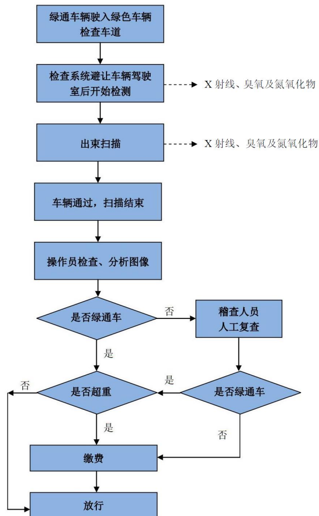
图 2-11 工作流程示意图及产污环节
