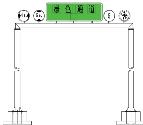
图 2-6 绿色通道入口龙门架示意图
