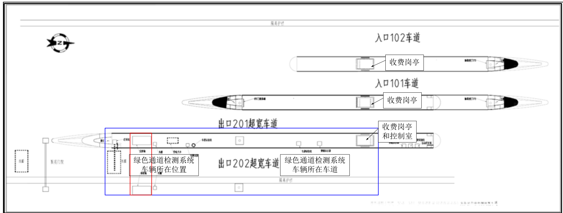
图 2-2 鸳鸯收费站 202 通道绿色通道车辆检查系统布置图
