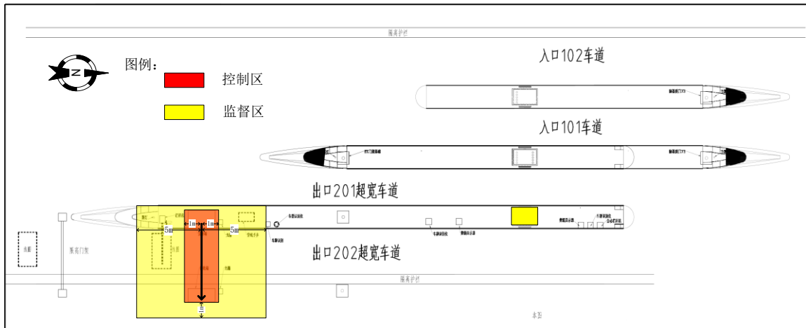
图 3-1 本项目辐射防护分区示意图
